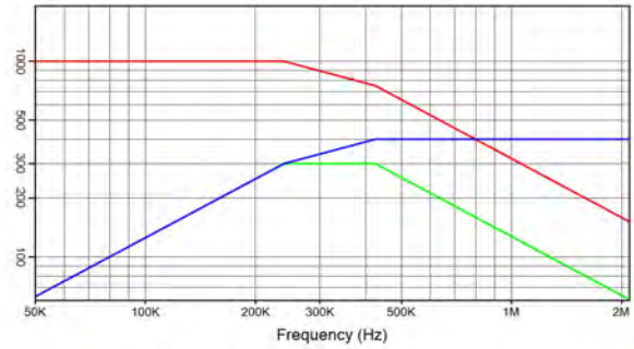
CSM 300N 0.2 \mu F 1000 V_{rms} 400 A_{rms} 300 kVA_r I(A) — Q( kVA_r ) — V_{rms} —
