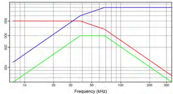
CSM 300N 5 \mu F 500 V_{rms} 800 A_{rms} 300 kVA_r I(A) — Q( kVA_r ) — V_{rms} —
