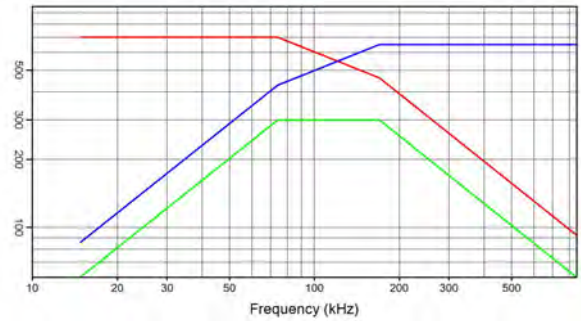
CSM 300N 1.32 \mu F 700 V_{rms} 650 A_{rms} 300 kVA_r I(A) — Q( kVA_r ) — V_{rms} —
