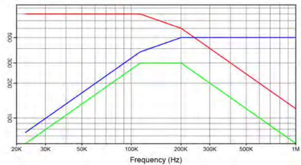
CSM 300N 0.66 \mu F 800 V_{rms} 500 A_{rms} 300 kVA_r I(A) — Q( kVA_r ) — V_{rms} —
