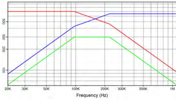
CSM 300N 1 \mu F 700 V_{rms} 650 A_{rms} 300 kVA_r I(A) — Q( kVA_r ) — V_{rms} —
