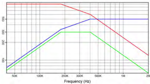
CSM 300N 0.33 \mu F 900 V_{rms} 500 A_{rms} 300 kVA_r I(A) — Q( kVA_r ) — V_{rms} —
