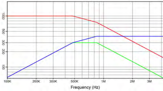
CSM 300N 0.1 \mu F 1000 V_{rms} 400 A_{rms} 300 kVA_r I(A) — Q( kVA_r ) — V_{rms} —
